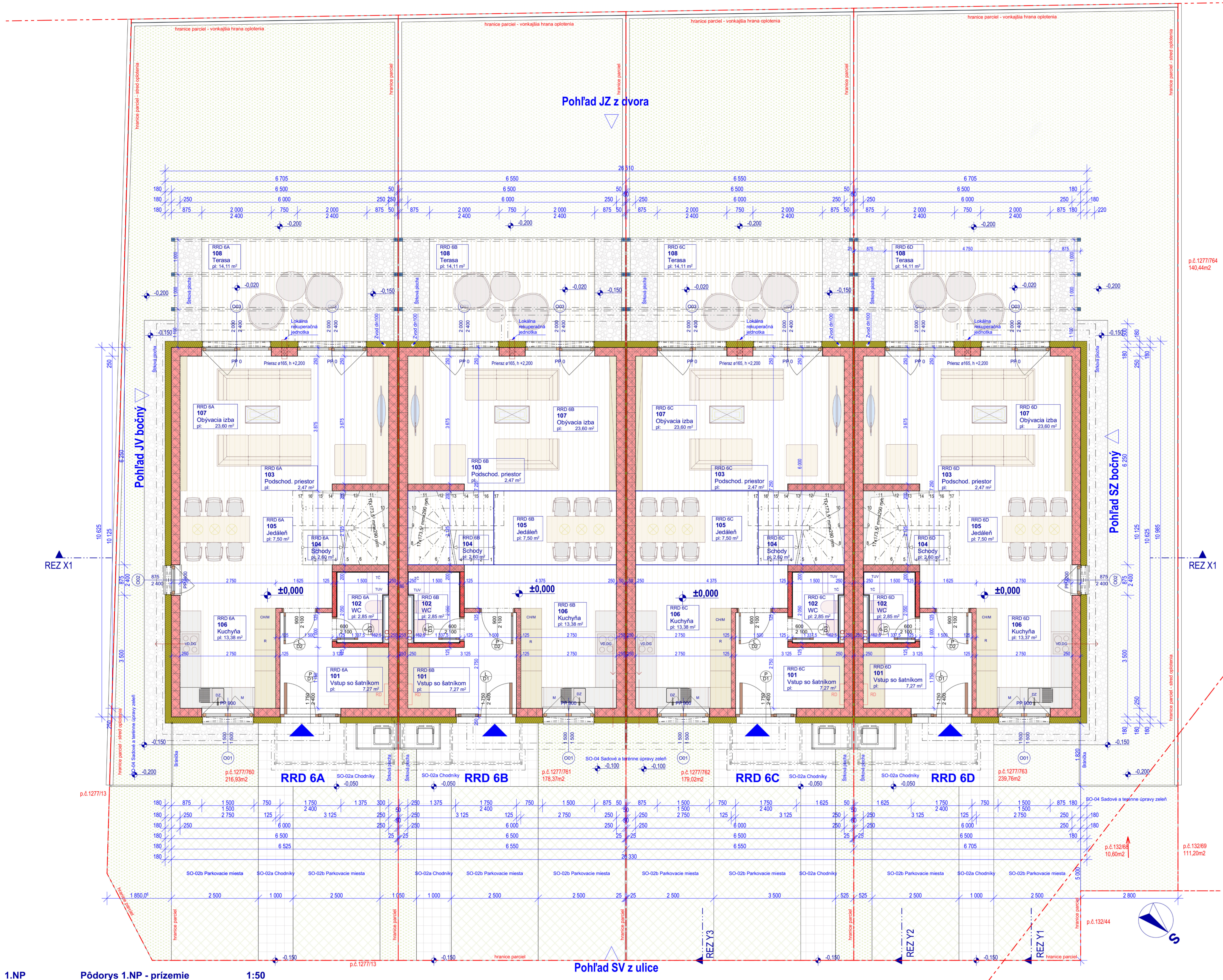
1.NP Pódorys 1.NP - prizemie 1:50
